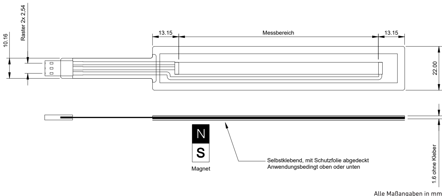
Alle Maßangaben in mm
