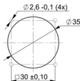
Einbau/Montageausschnitt
